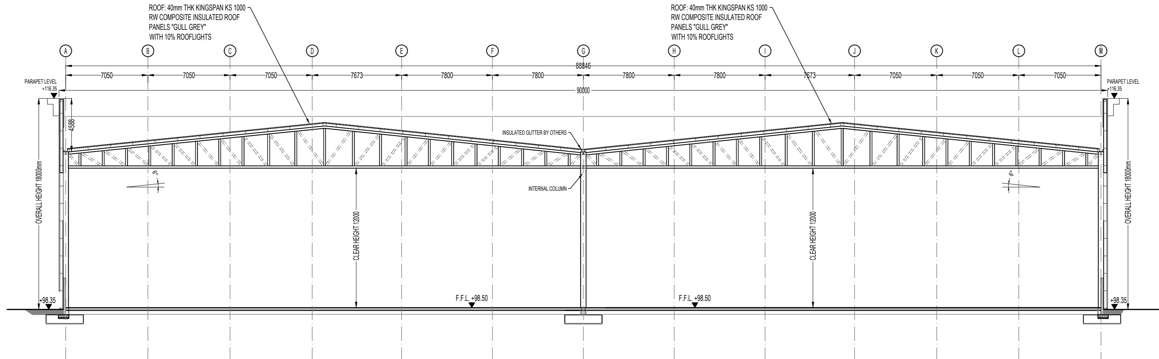
SECTION A-A SCALE 1:200
